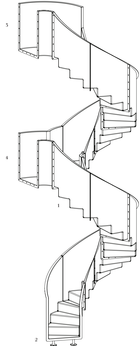
Constructed Elementstair (5 floor example) Elementstair-constructie (voorbeeld met 3 verdiepingen)
